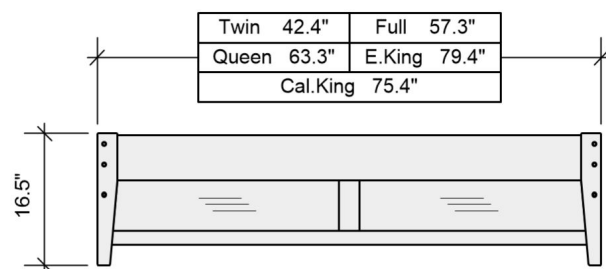
Basic Footboard (KPF)
